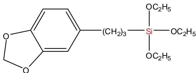
SiSiB ® PC9922 Tert-butylcyclopentadienyltrimethylsilane N.A.
